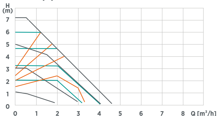
Charakterystyka WITA Delta MAXI 70
