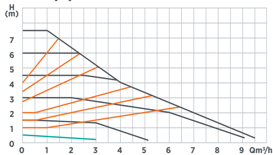
Charakterystyka WITA Delta HE 75 F
